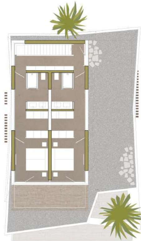
UPPER FLOOR / PLANTA ALTA
