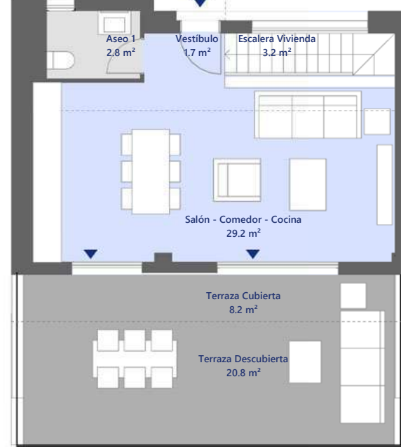
Planta primera
