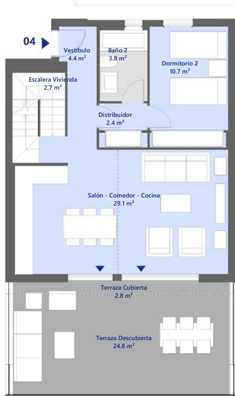
Planta baja
