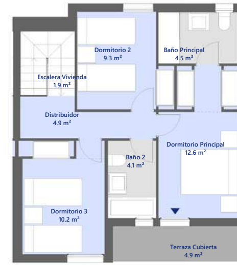
Planta primera
