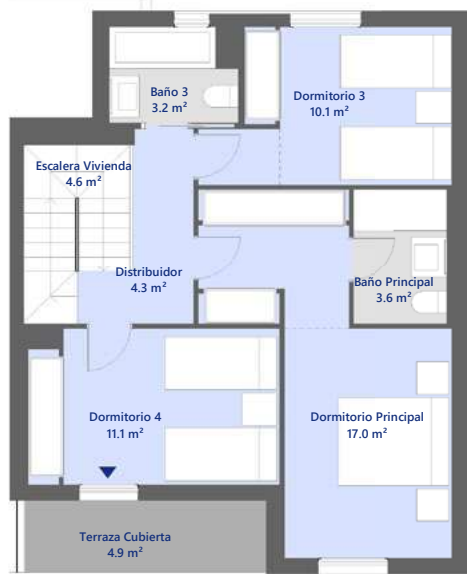
Planta primera
