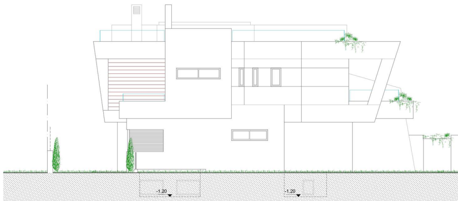
Alzado Lateral
