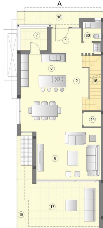
PLANTA BAJA
