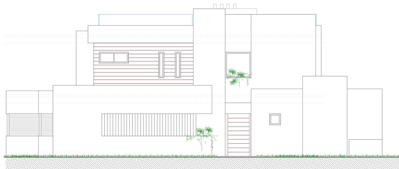
ALZADO ENTRADA
