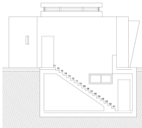
ALZADO LATERAL SUR
