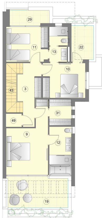
PLANTA PRIMERA
