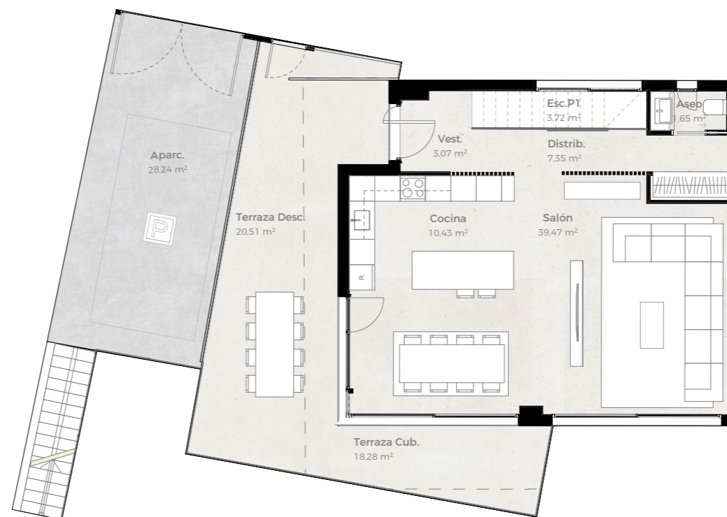
PLANTA PRIMERA
