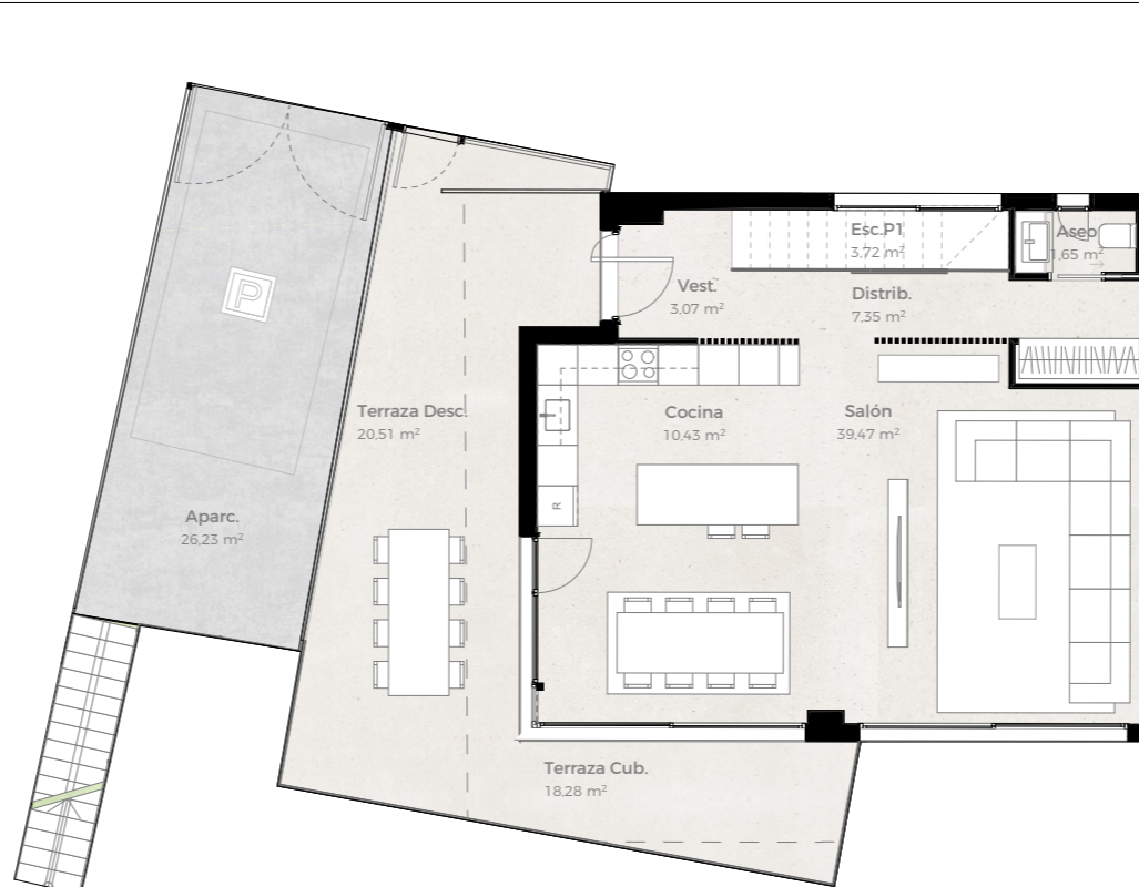
PLANTA PRIMERA
